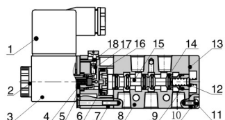
4V320
