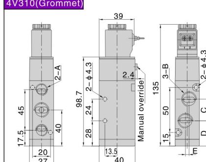
4V310(Grommet)
