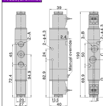
4V320(Grommet)
