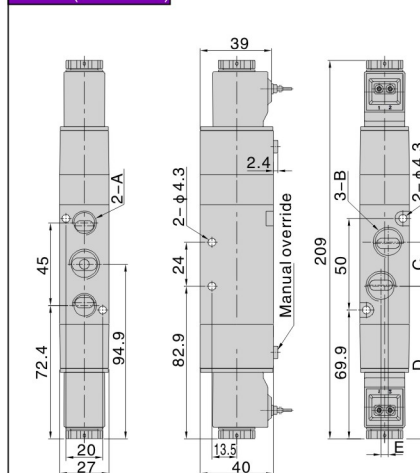
4V330(Grommet)
